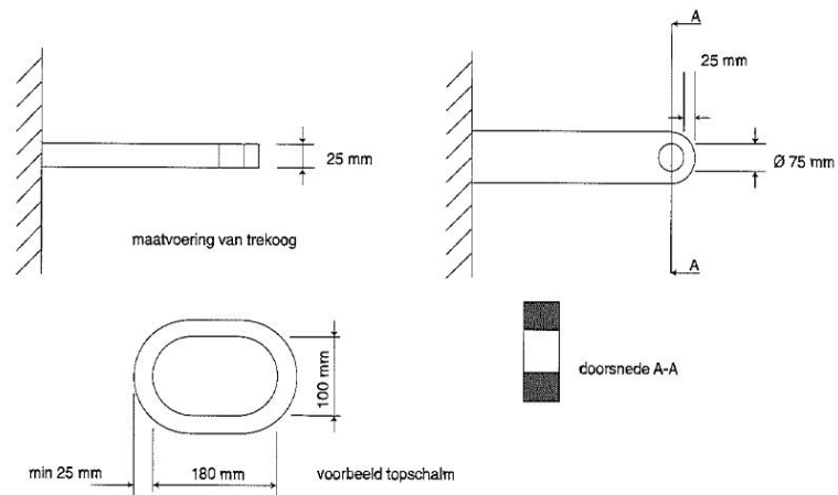
Figuur 32: maatvoering trekoog en topschalm
