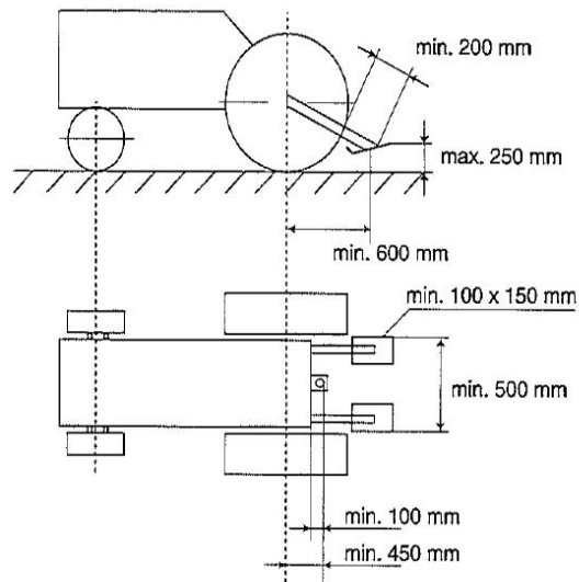
Figuur 31: constructie/maatvoering steigerbegrenzer
